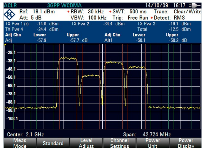
采用4载波测量 3GPP WCDMA 信号的邻道泄漏比 (ACLR)。
